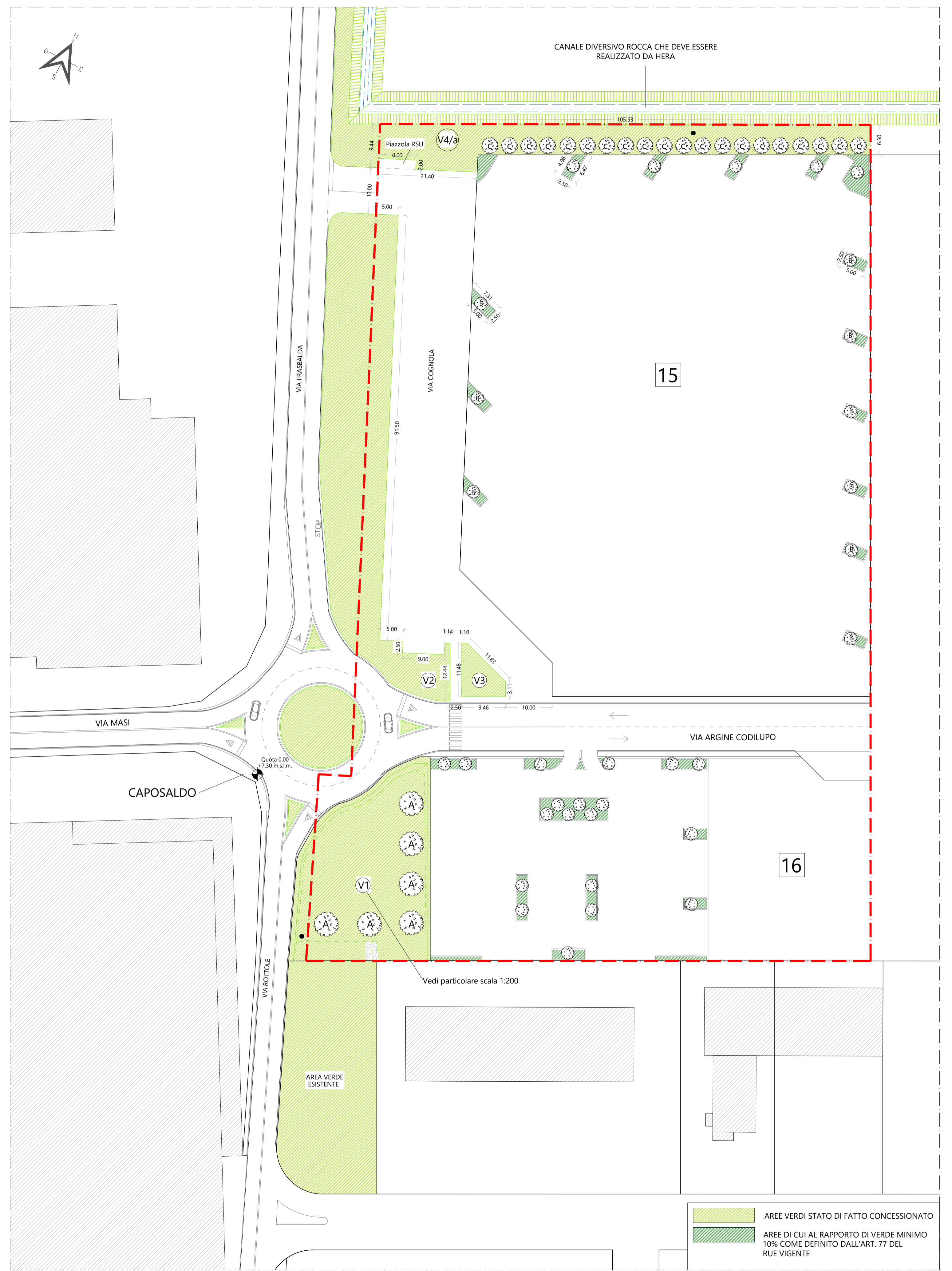
STATO DI FATTO CONCESSIONATO E PROGETTO DI VARIANTE AREE VERDI (1:500)
