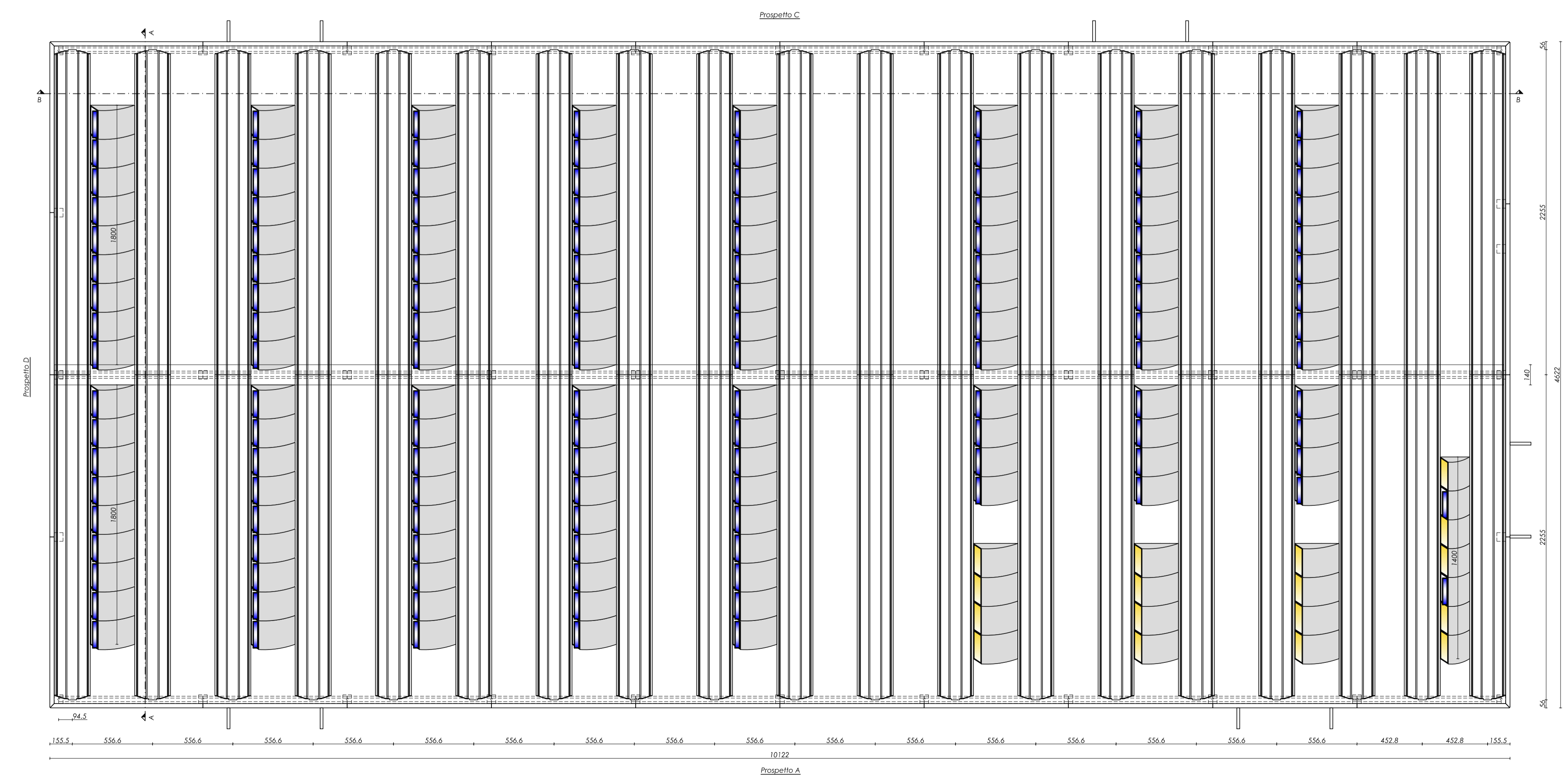
PIANTA COPERTURA
